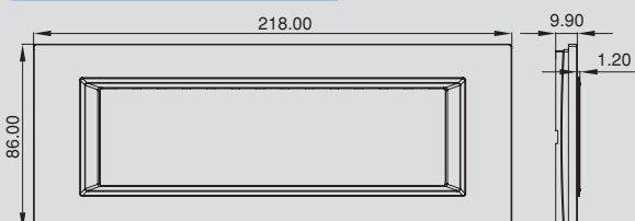
Ultima 7M Frame
