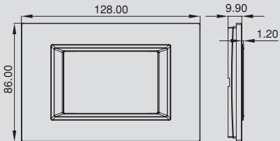
Ultima 3M Frame
