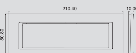
Optima 7M Frame
