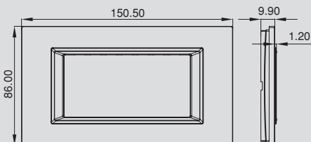
Ultima 4M Frame
